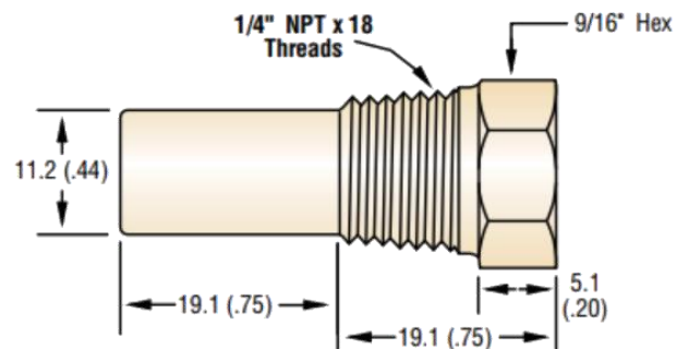
Style 117 1000 p.s.i.
